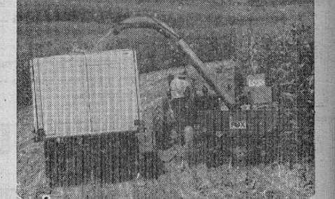
Una cosechadora, de fabricación estadounidense, se ve en funcionamiento en una granja del Estado de Maryland. La máquina corta el maíz, desmenuza los tallos, y fuerza el estiraje a través del tubo hacia el camión que va a su lado. Almacenado en un silo, el ensilaje sirve como forraje de invierno para el ganado de la granja.
